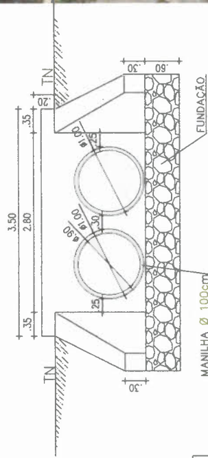
02 VISTA LATERAL ESCALA: 1 / 50
